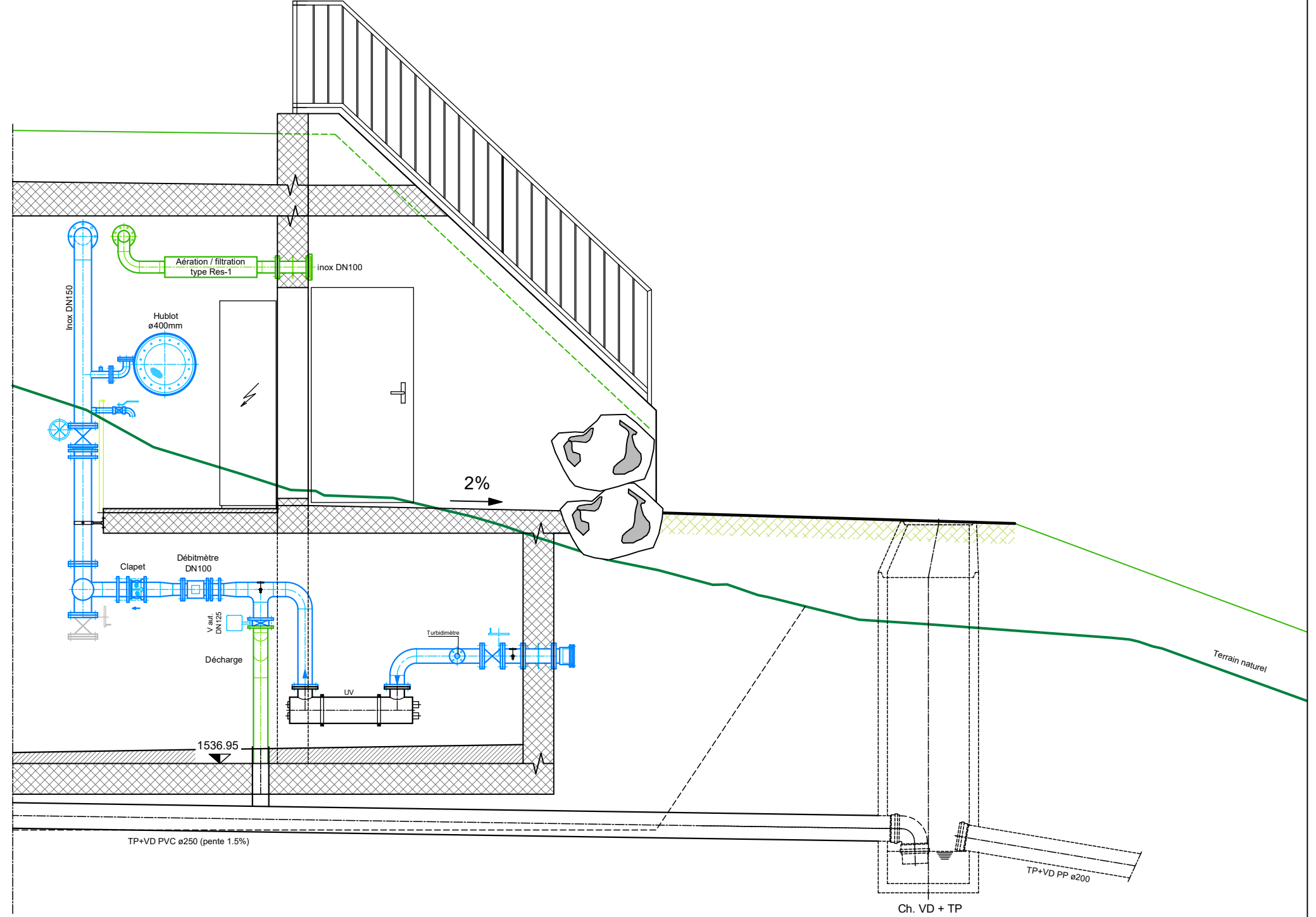
Détail désinfection UV
