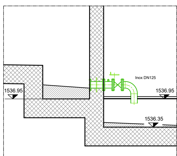
Détail vidange
