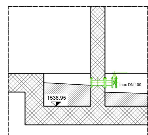
Détail vidange
